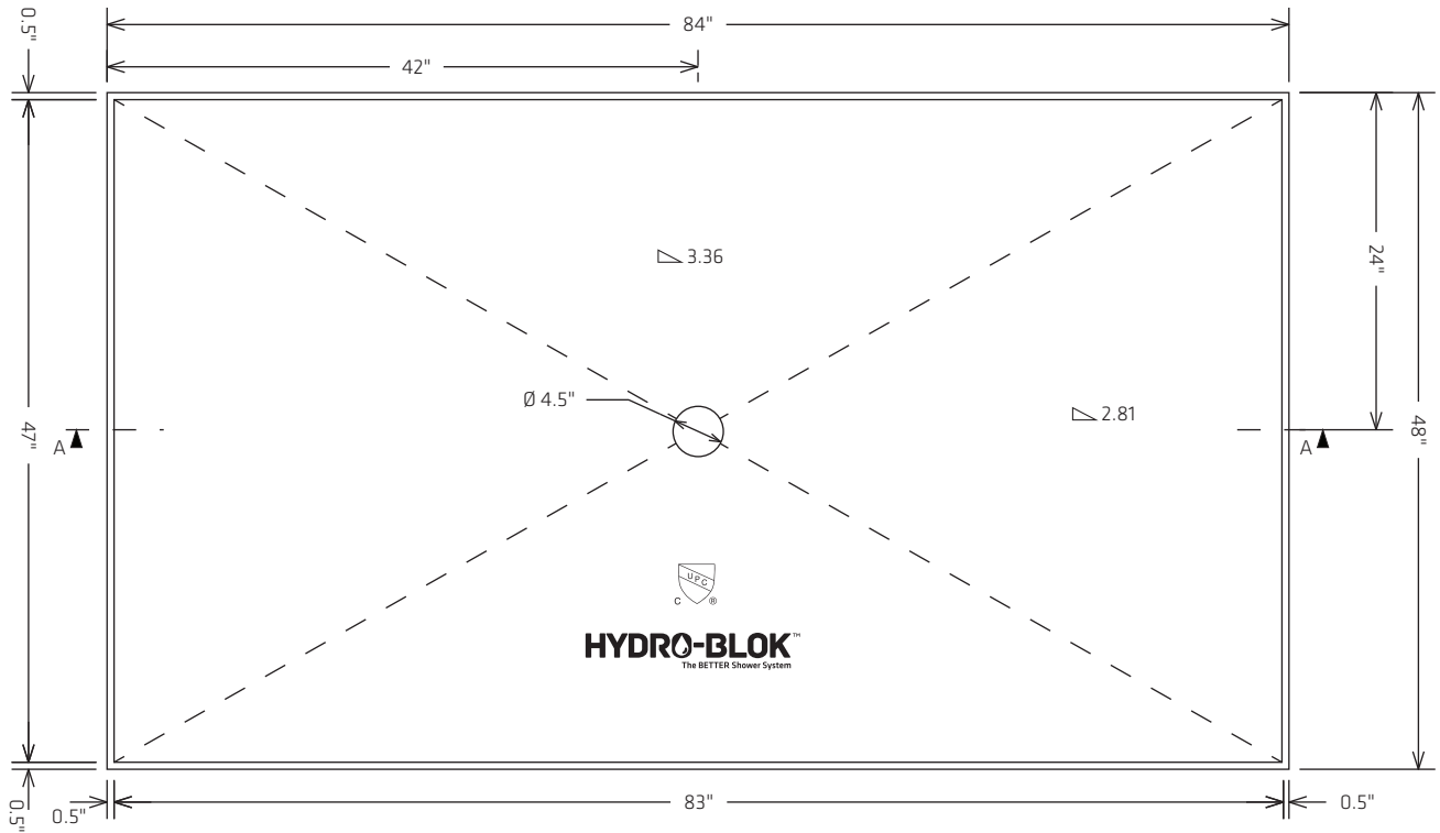
Section A-A
